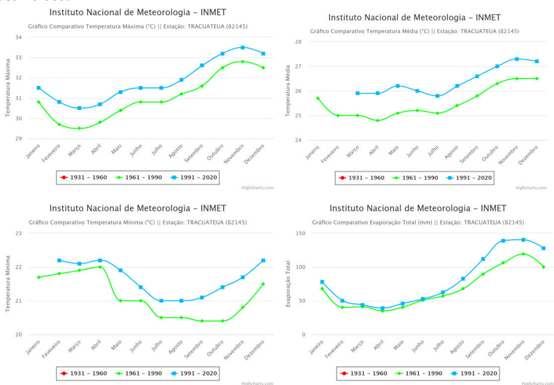
Figura 28 - Dados Meteorológicos da Estação Convencional de Traquateua para a Temperatura Máxima, Temperatura Média, Temperatura Mínima, Evaporação e precipitação acumulada.
