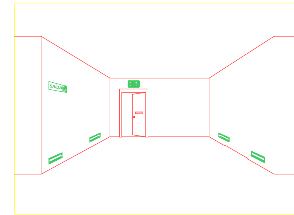
DET. SINALIZAÇÃO DE SAÍDA SOBRE PORTA CORTA-FOGO SINALIZAÇÃO COMPLEMENTAR DE SAÍDAS E OBSTÁCULOS SEM ESCALA
