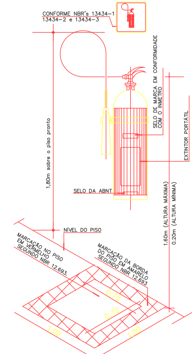
DET 01 - EXTINTOR S/ ESC.
