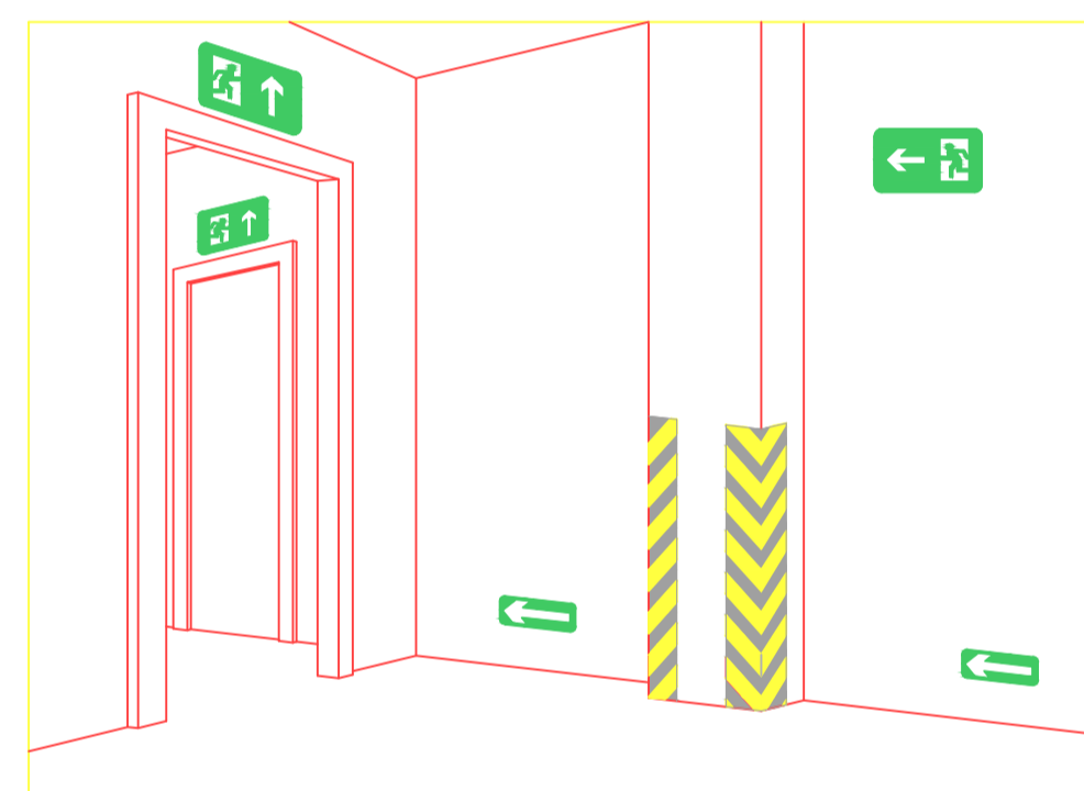
DET. SINALIZAÇÃO DE SAÍDA SOBRE VERGAS DE PORTAS SINALIZAÇÃO COMPLEMENTAR DE SAÍDAS E OBSTÁCULOS SEM ESCALA
